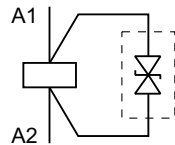
Transil diode
